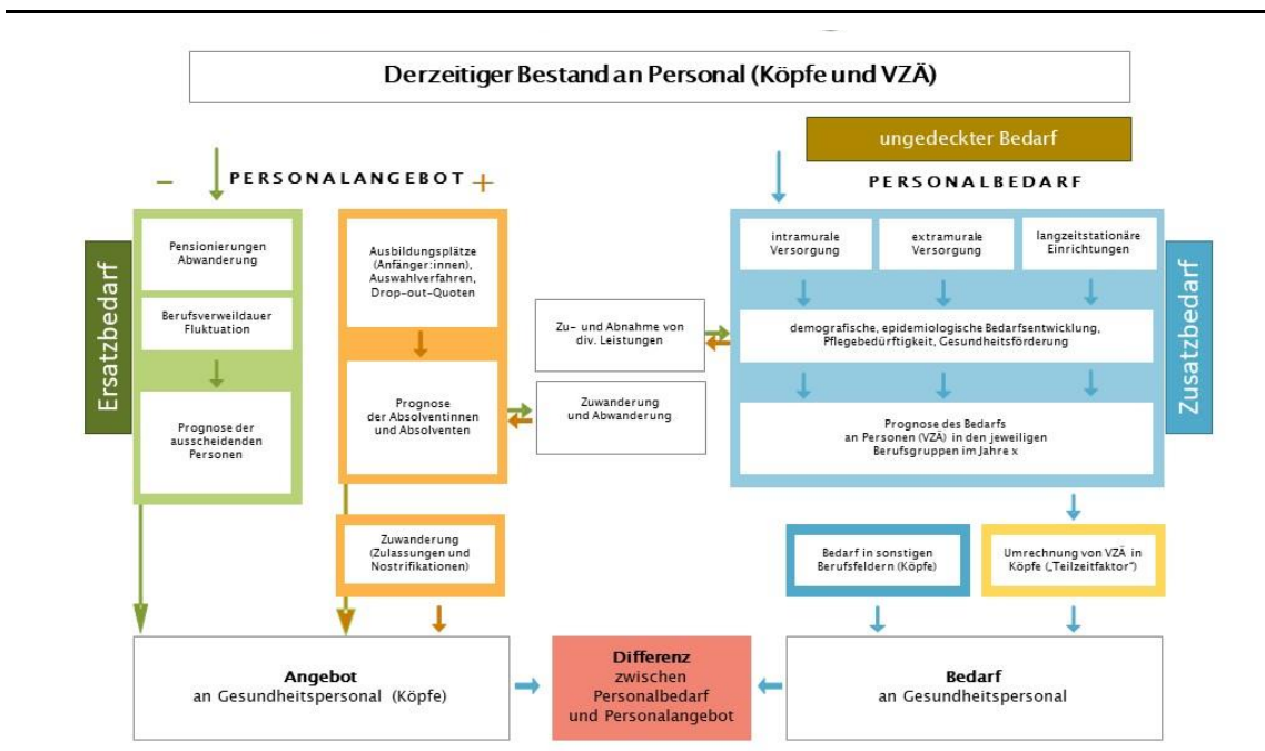
Abbildung 6.1: Prognosemodell zur Personalbedarfsplanung
