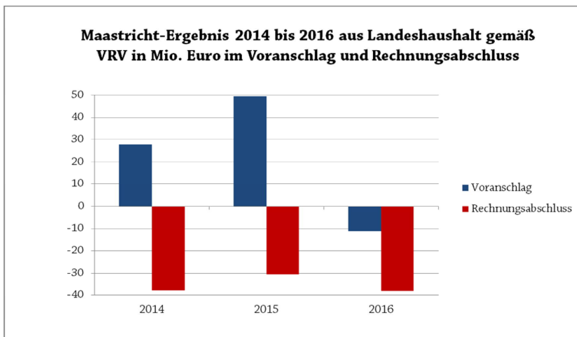
Abbildung 17: Maastricht-Ergebnis 2014 bis 2016
