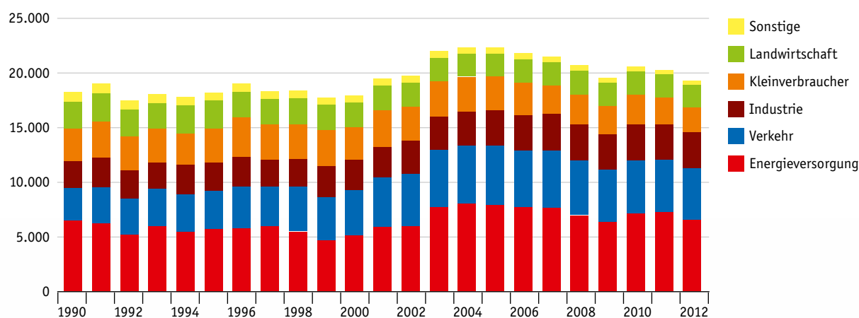
Abb. 14 Treibhausgasemissionen NÖ – 1990–2012 in kt CO 2 eq
