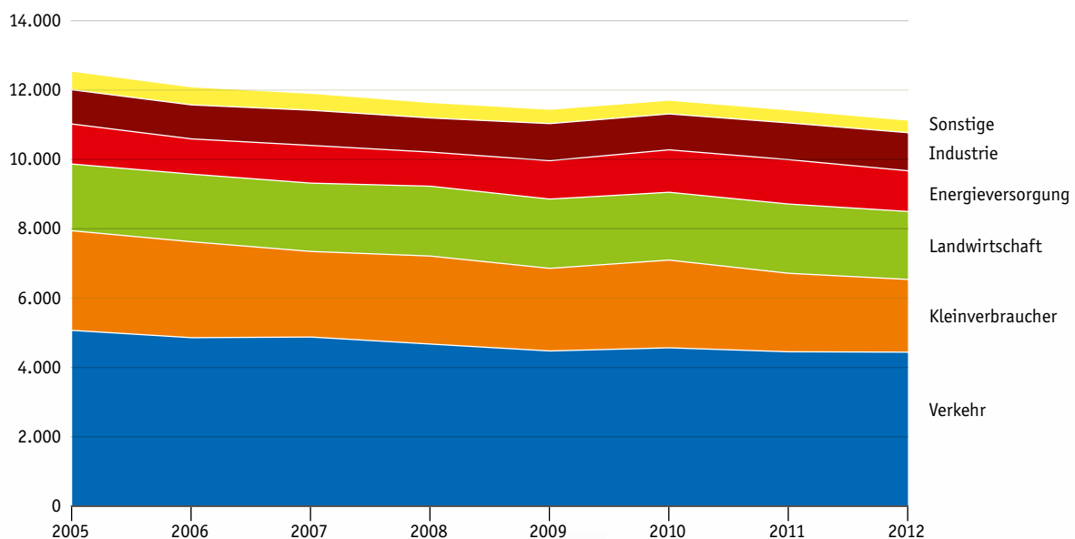
Abb. 10 Treibhausgasemissionen NÖ Nicht-ETS-Bereiche 2005–2012 (BLI)
