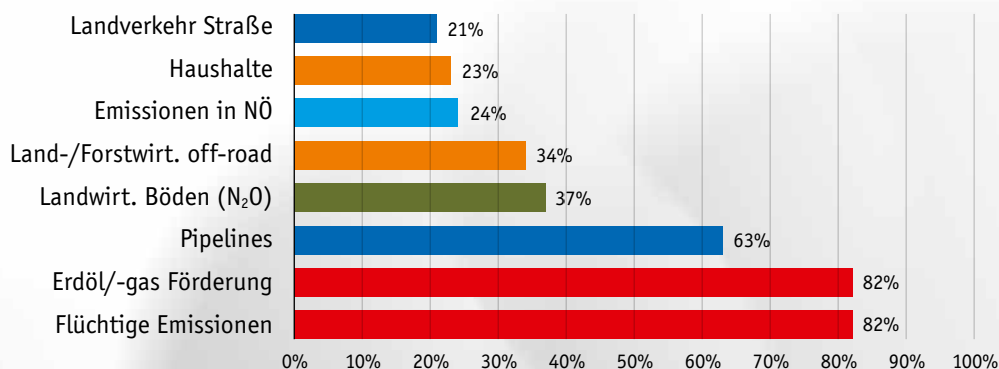
Abb. 13 NÖ-Anteil an nationalen Emissionen
