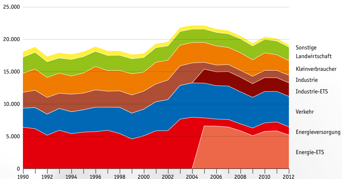
8 Treibhausgasemissionen NÖ 1990–2012 in kt CO 2 eq
