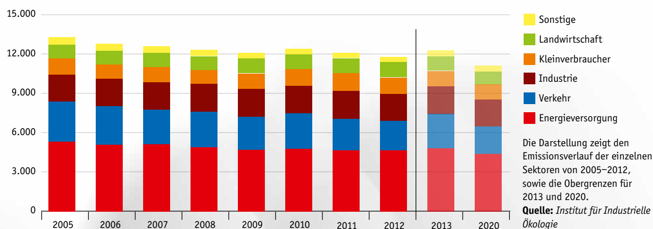
Abb. 15 Treibhausgasemissionen NÖ Nicht-ETS-Bereiche, Trend 2005–2012 und Basis 2013 & Ziel 2020 (BLI)
