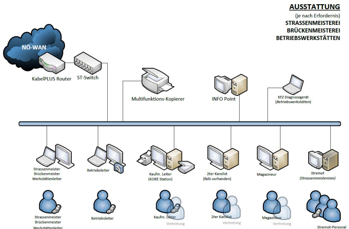
Abbildung 4: Ausstattung Straßen-, Brückenmeistereien und Betriebswerkstätten
